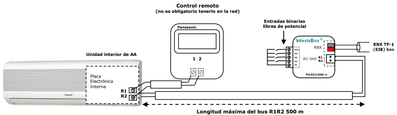
Figure 2.1 Diagrama de conexiones para PA-RC2-KNX-1i
