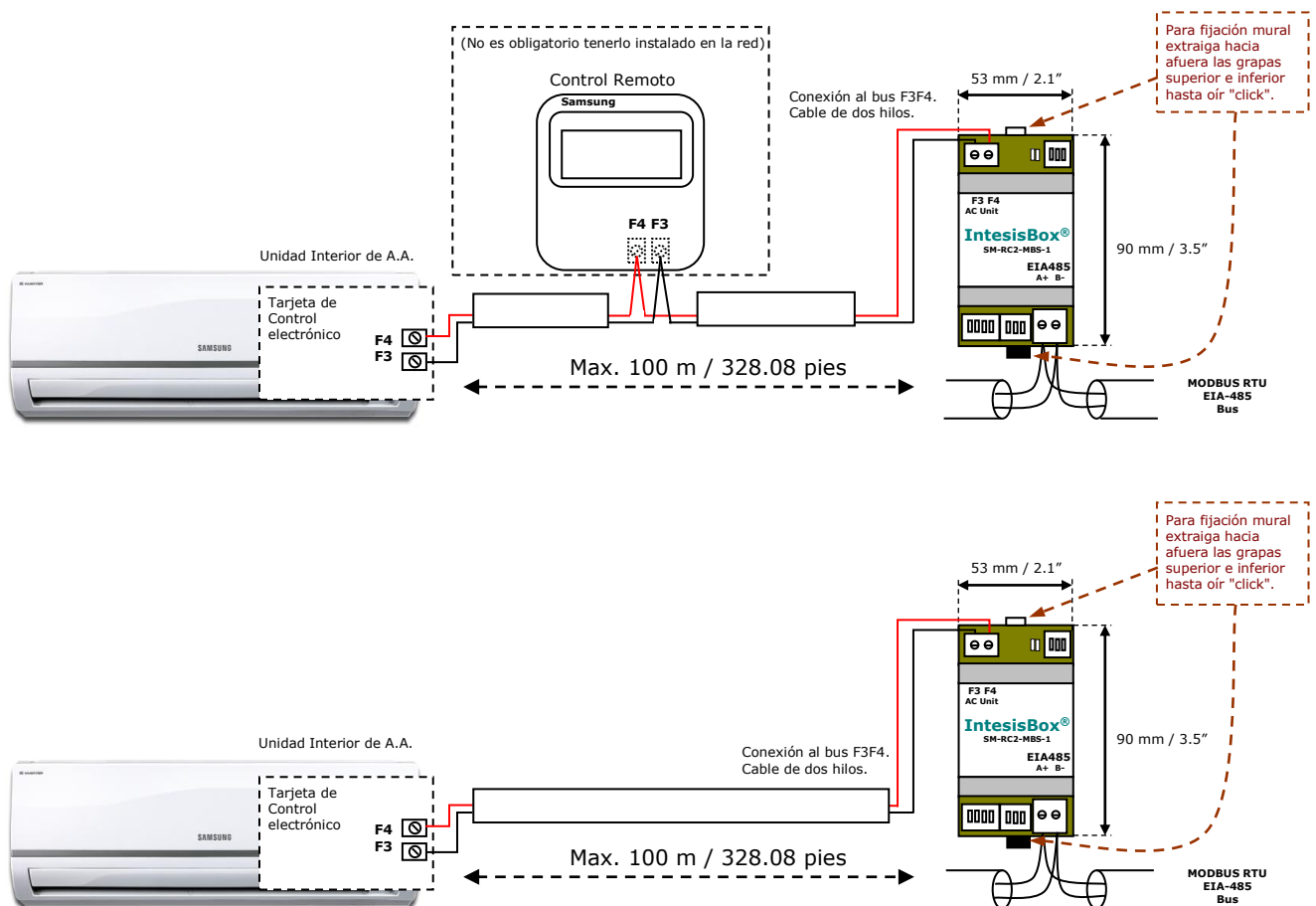
Figura 2. 1 Diagramas de conexión del SM-RC2-MBS-1
